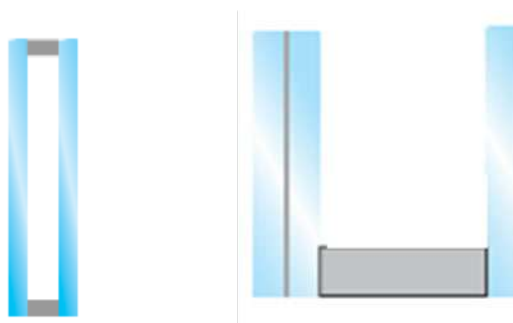
Figure 9 : schéma d'un vitrage isolant double de type 4/16/4 (à gauche) et 44.2/12/4 (à droite)
